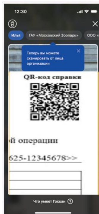
Рисунок 36 – Проверка QR-кода
